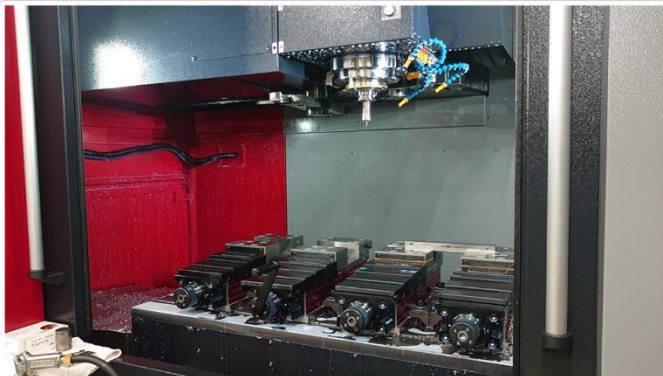
部品の機械加工
